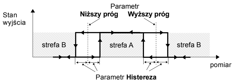
Rys. 7.89. Sterowanie dwuprogowe wyjścia przekaźnikowego
