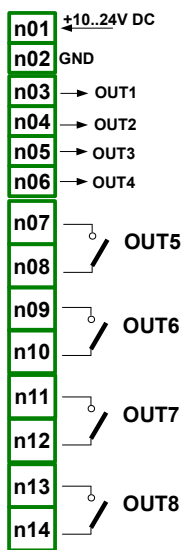
Rys. 8.12. Mieszane moduły wyjść przekaźnikowych
