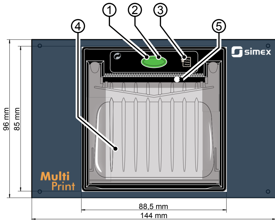
Rys. 8.19. Widok płyty czołowej
