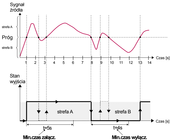
Rys. 7.92. Zasada pracy wyjść przełącznikowych dla przykładowych ustawień czasowych: Min.czas załącz. = 5 sec., Min.czas wyłącz. = 4 sec.
