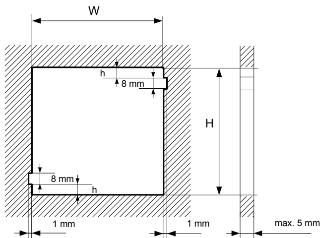
Rys. 4.2. Wymiary montażowe
