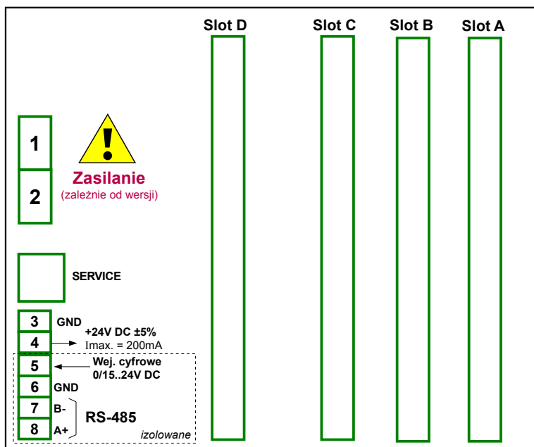
Rys. 4.8. Opis wyprowadzeń
