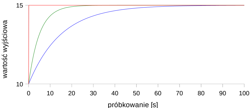
Rys. 7.52 Przykładowy przebieg sygnału wejściowego (wykres czerwony) oraz sygnał przetworzony dla w=5 (wykres zielony) i w=15 (wykres niebieski)
